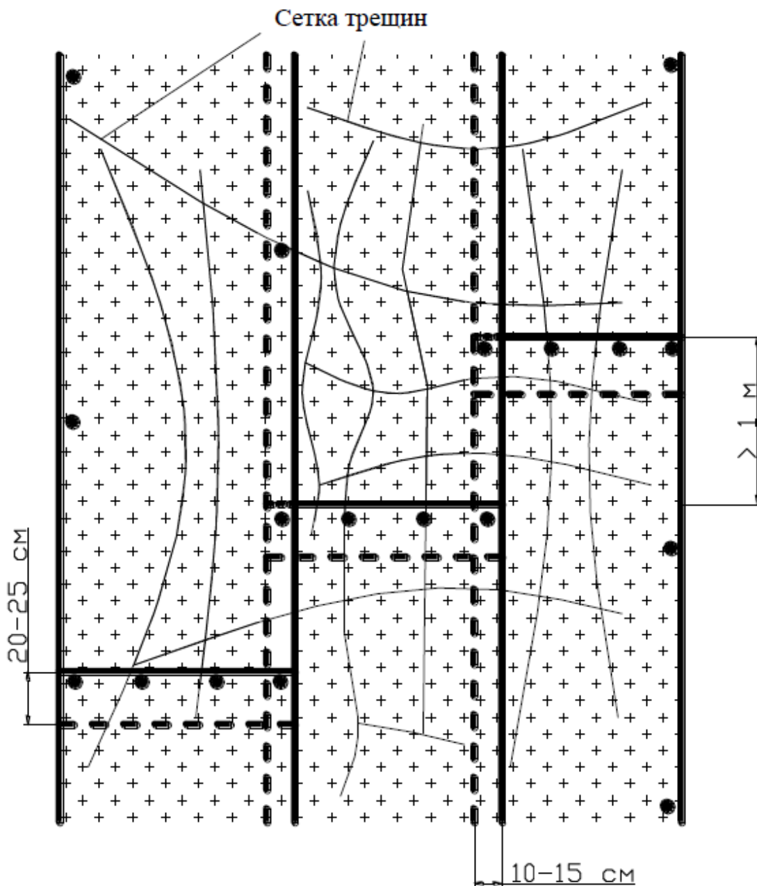
Рисунок 8 – Схема сплошного армирования геосеткой
