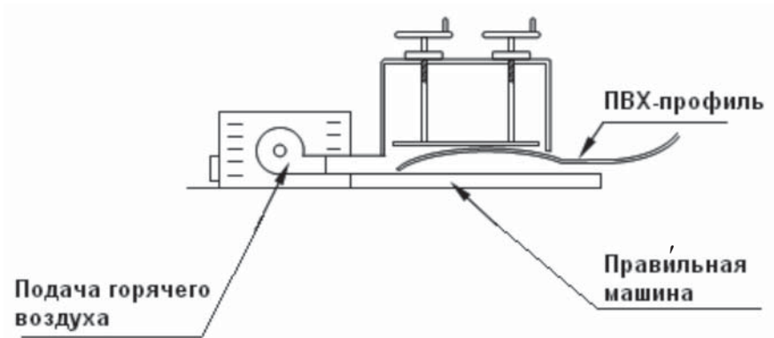
Рисунок К.2 – Правка конца профиля
