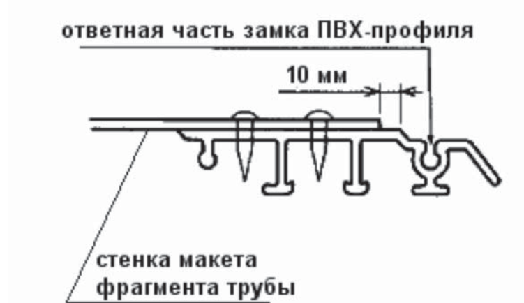
Рисунок 6 – Фиксация кольца из ПВХ-профиля в макете фрагмента трубы
