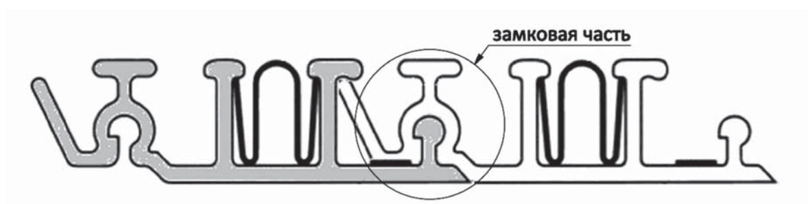
б) Способ скрепления витков профиля между собой
