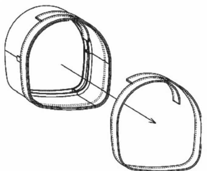
Рисунок 5 – Навивка кольца из профиля на макет трубы
