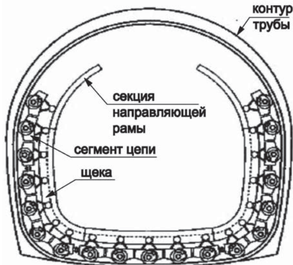
Рисунок 9 – Третий этап сборки навивочной машины
