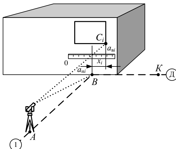
Рисунок В.2 – Метод наклонного проектирования
