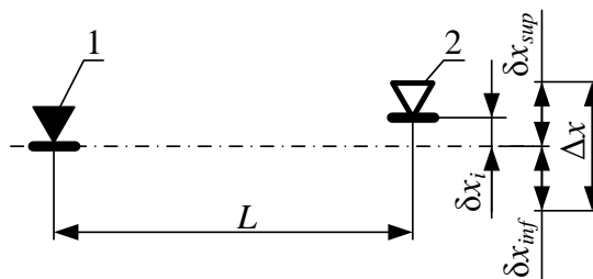
Рисунок 10 – Допуск и отклонение разбивки высотных отметок
