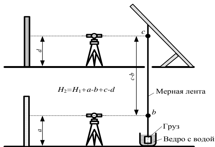
Рисунок Б.8 – Схема передачи отметки на монтажный горизонт
