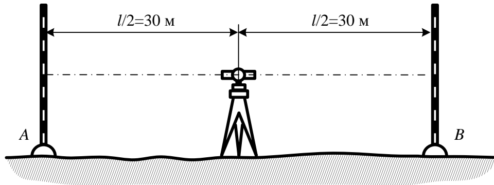
Рисунок Д.1 – Первая конфигурация хода для упрощенной методики испытания
