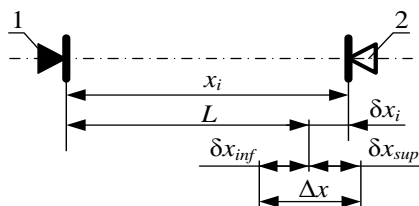
Рисунок 7 – Допуск и отклонение разбивки точек и осей в плане
