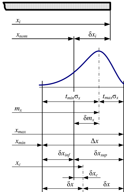
Рисунок Г.1 – Схема взаимосвязи характеристик точности при несимметричном распределении геометрического параметра
