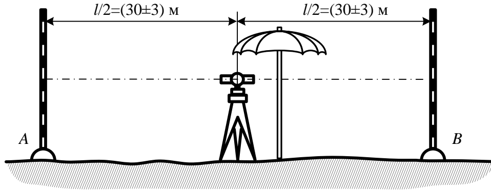
Рисунок Д.3 – Конфигурация хода для полной методики испытания
