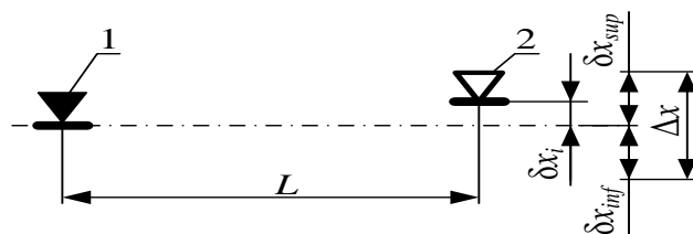
Рисунок Б.1 – Схема допусков и отклонений передачи высотных отметок
