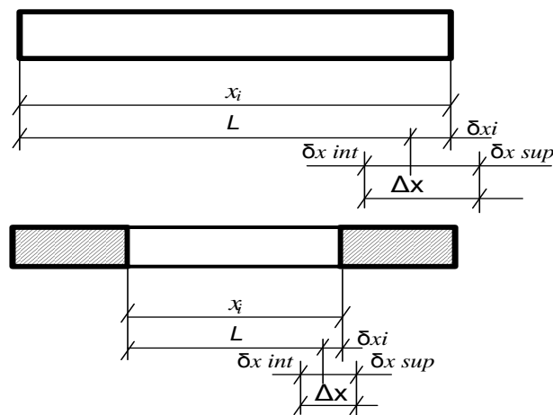
Рисунок 1 – Допуск и отклонение от линейных размеров элементов
