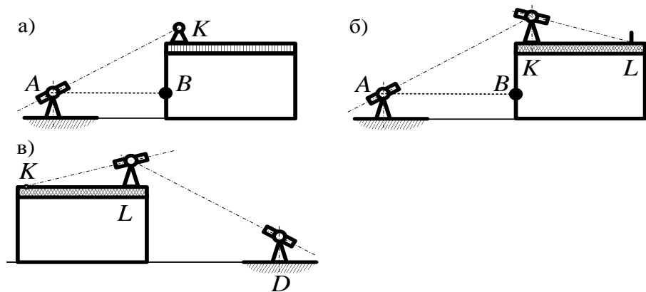
Рисунок Б.7 – Определение положения оси на монтажном горизонте
