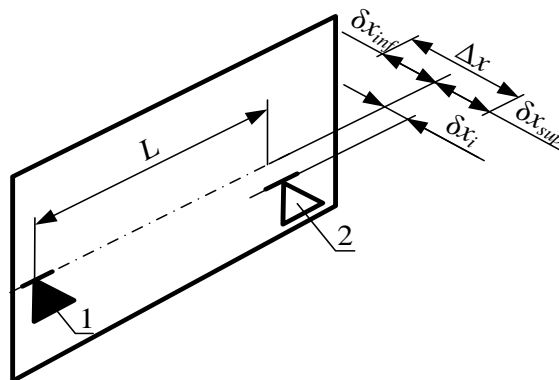
Рисунок Б.2 – Схема допусков и предельных отклонений при передаче точек и осей по вертикали
