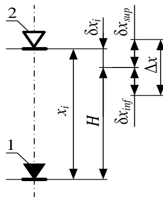
Рисунок Б.3 – Схема допуска створности и отклонения от створности точек
