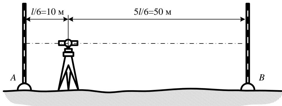
Рисунок Д.2 – Вторая конфигурация хода для упрощенной методики испытания
