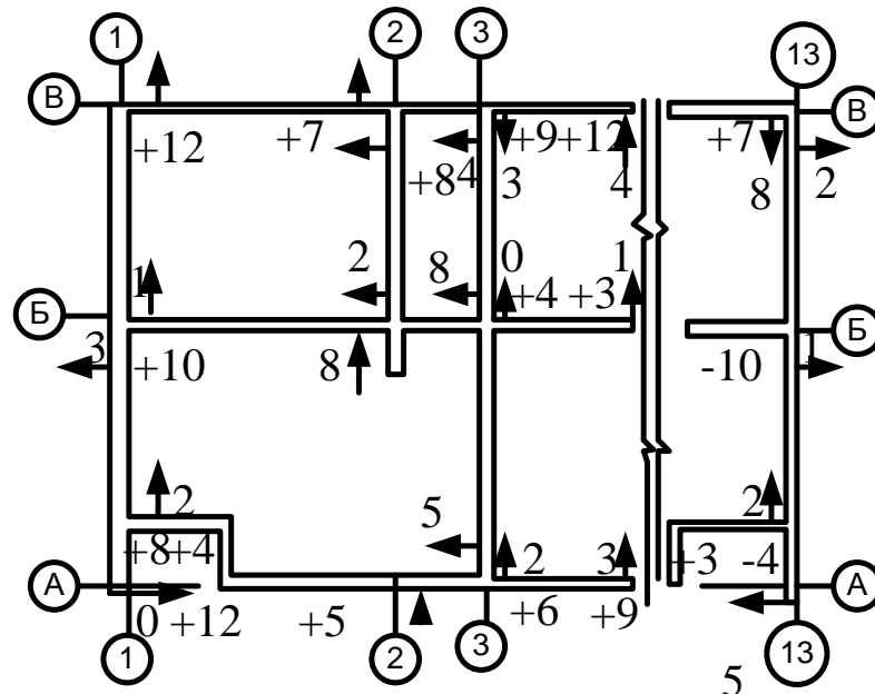
Рисунок П.2 – Пример исполнительной схемы планово-высотного положения стаканов фундаментов под железобетонные колонны
