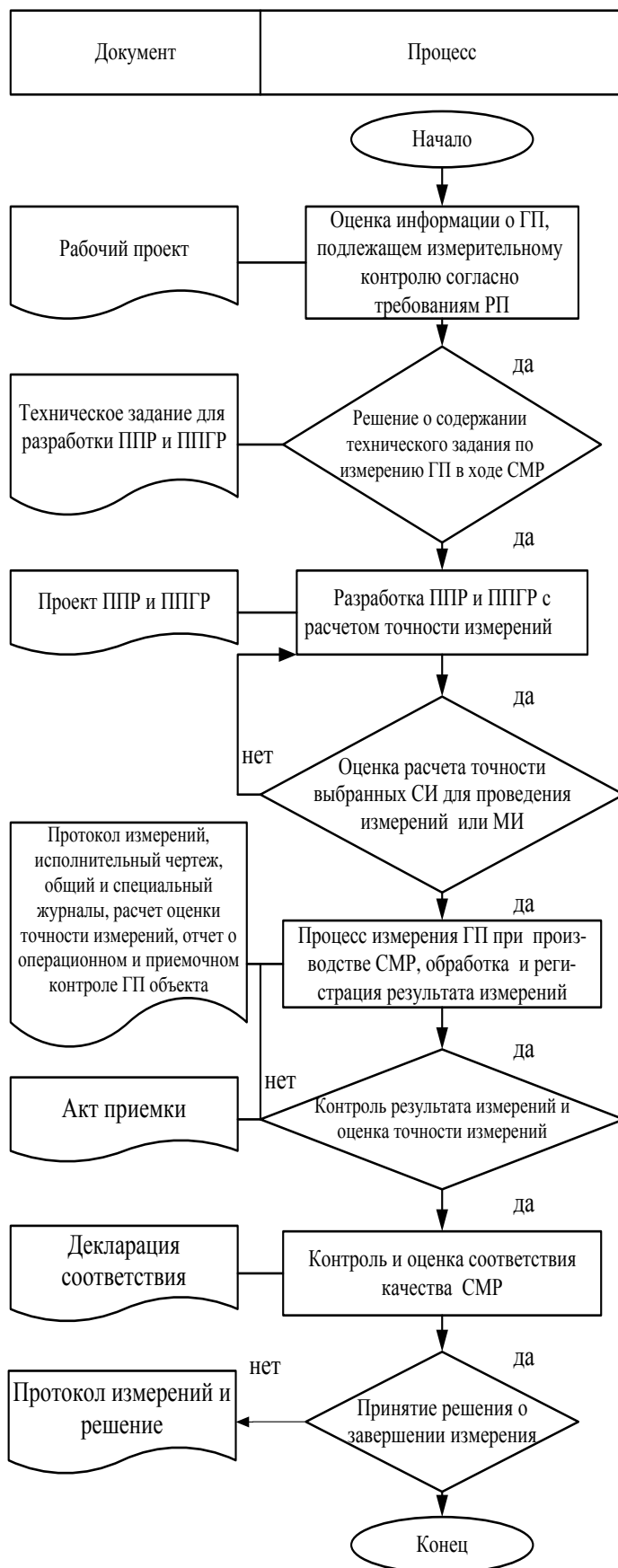
Рисунок 13 – Схема процесса измерений геометрических параметров – расширенная неопределенность U .
