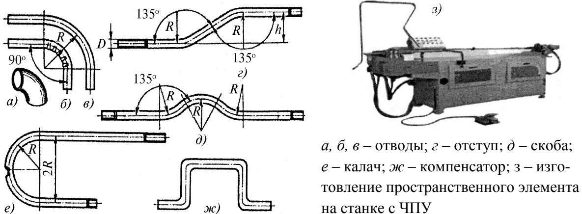
Рисунок 7.1 – Гнутые детали трубопроводов
