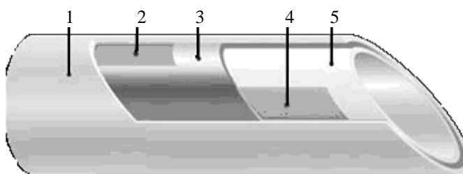
Рисунок 5.10 – Металлополимерная труба
