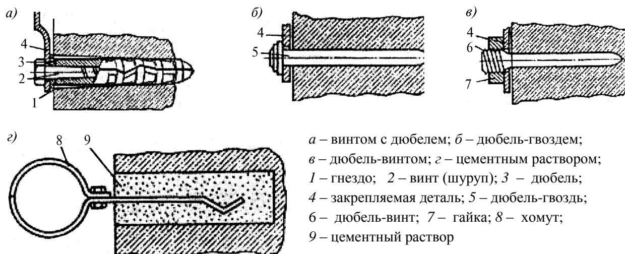
Рисунок 8.5 – Установка крепежа водопроводов в строительных конструкциях
