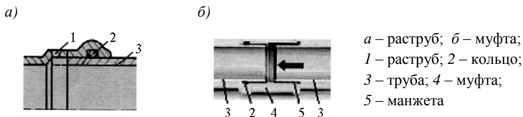
Рисунок 6.18 – Соединения канализационных труб из наполненного полипропилена
