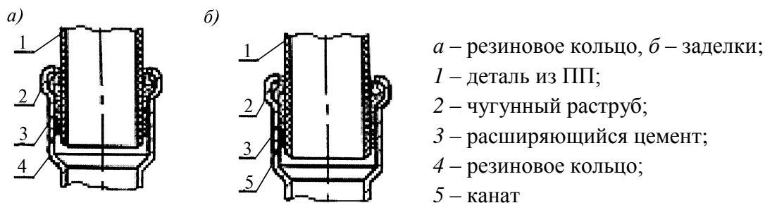
Рисунок 6.17 – Раструбные соединения труб из ПП с чугунными трубами
