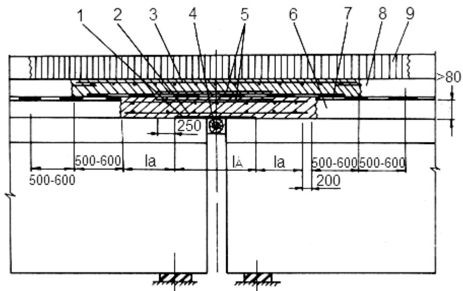
Рисунок 7.3 Схемы объединения пролетных строений в температурно-неразрезные
