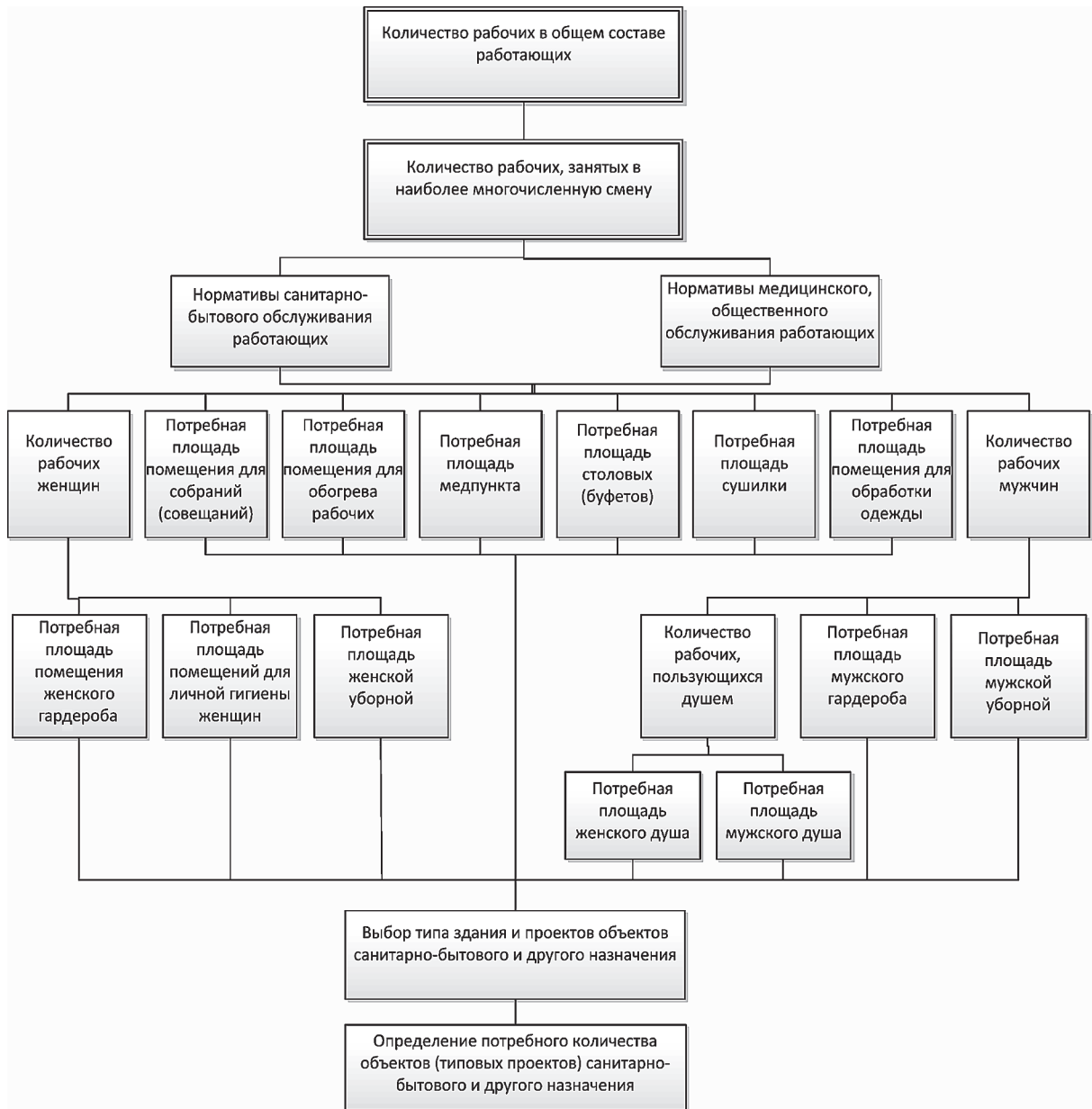
Рисунок 3 – Последовательность расчета потребности в мобильных зданиях
